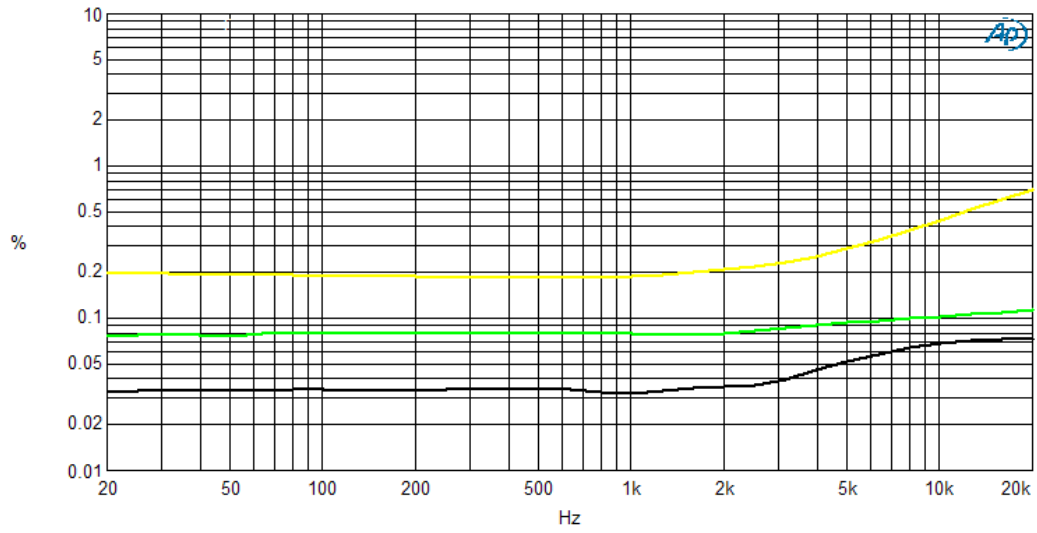
T.H.D.+N vs. frequency @ 8Ω (1W black, 10W green, 150W yellow) T.H.D + N rispetto alla frequenza su 8Ω ( 1W curva nera, 10W curva verde e 150W curva gialla)
