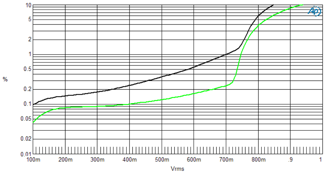
T.H.D.+N vs. Input Amplitude @ 8Ω (20kHz black, 1kHz green) T.H.D + N rispetto alla tensione di ingresso su 8Ω ( 20kHz curva nera, 1kHz curva verde)
