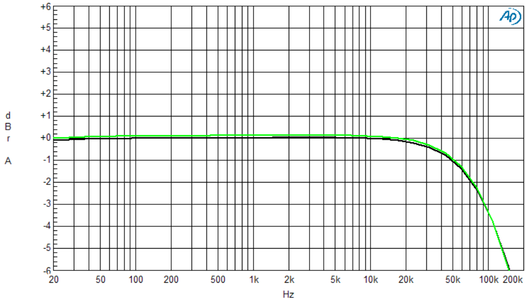
1W frequency response right plus left channel - Risposta in frequenza ad 1W canale destro e sinistro
